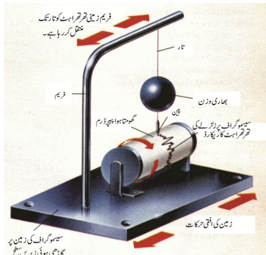
سیسموگراف
